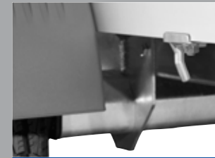
Ergots de sanglage vissables (option)
